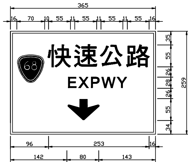
註 快速公路之英譯採「EXPWY」縮寫設計。
