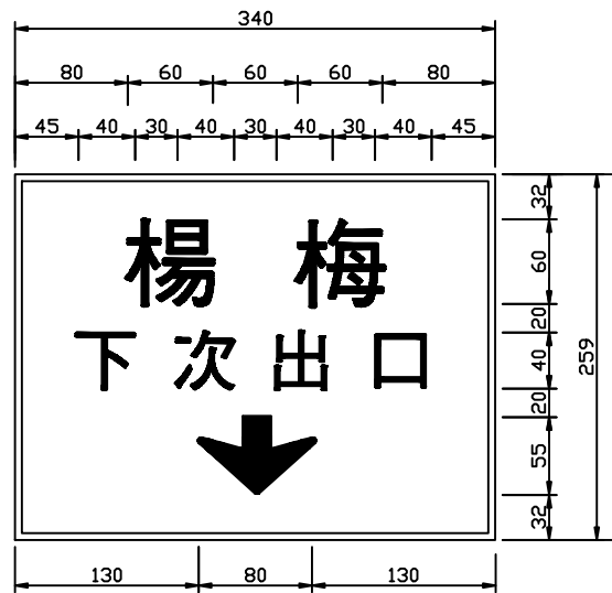
註：適用於「下次出口」之車道指示標誌。
