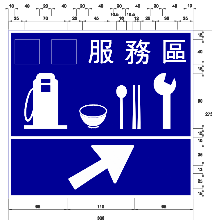
高速公路服務區進口方向標誌 (W-W/BL)
