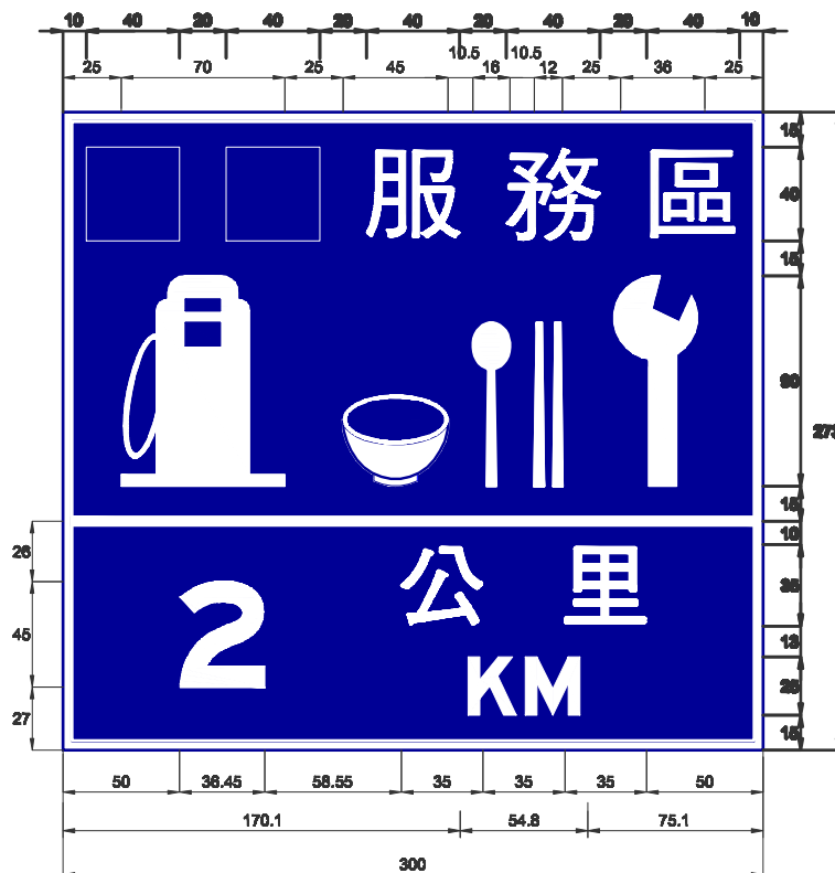
高速公路服務區預告標誌 (W-W/BL)
